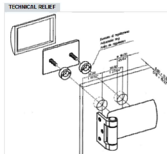
Hinge Millig & Positioning Art. Nr. 350.40.956.00
